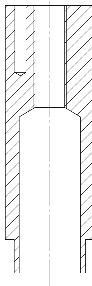
SECTION A-A SCALE 1.5 : 1
